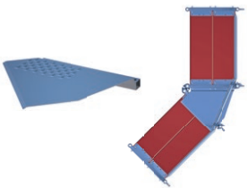
Echbelag flexibel, 2-bohlig Art.-Nr. 00678
